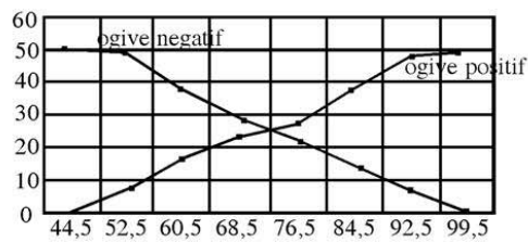
Gambar 1.6 Ogive negatif dan ogive positif
