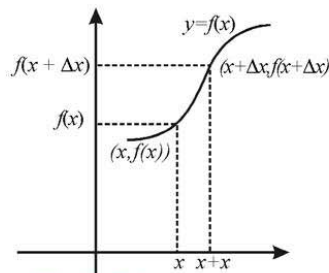
Gambar 5.1 Taksiran geometri turunan di titik y
