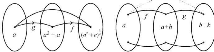
Gambar 5.2 Pendiferensialan fungsi komposisi f \circ g
